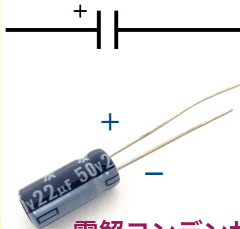
電解コンデンサ
